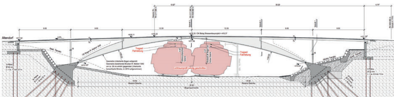
Abb. 6: Längsschnitt der neuen Brücke
