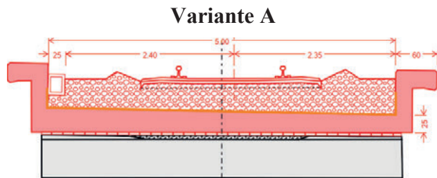
Abb. 2: Querschnitt Variante A: Stahlbeton-Schottertrog auskragend
