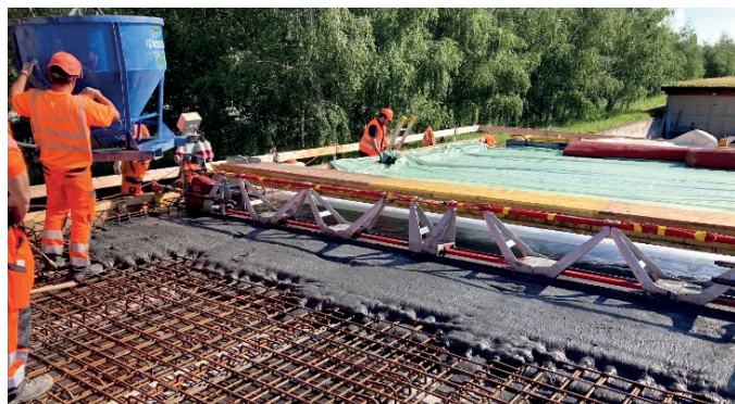
Fig. 18 : Mise en oeuvre CFUP type UB Tablier
