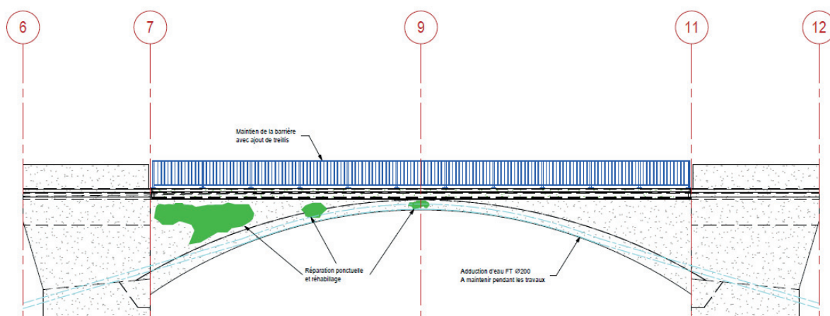
Fig. 3 : Vue en élévation du pont
