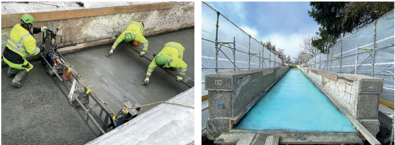
Abb. 14: Einbau des Belags in UHFB-Kiesmatrix Abb. 15: Verzögerer in blau als Nachbehandlung
