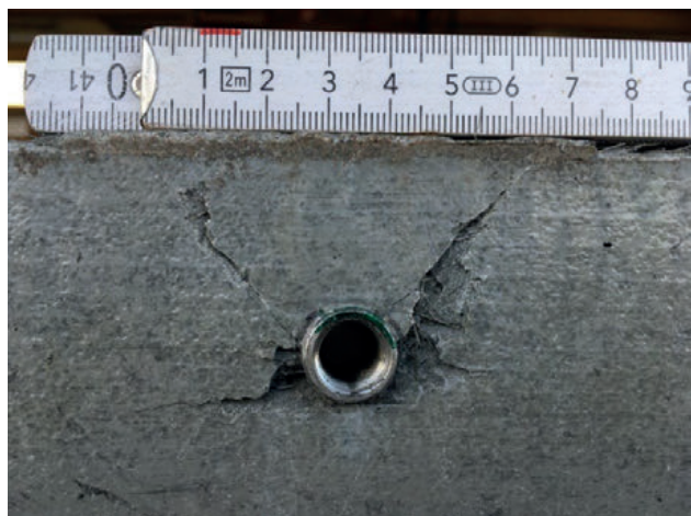
Abb. 21: Rissbild im UHFB bei Muffe M12 mit Gewindestab nach Versagen
