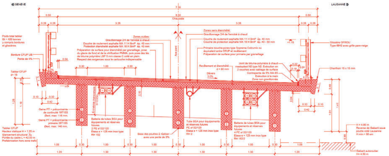
Fig. 7 : Coupe transversale – Epaisseur du tablier 150mm / Largeur des poutres 300mm
