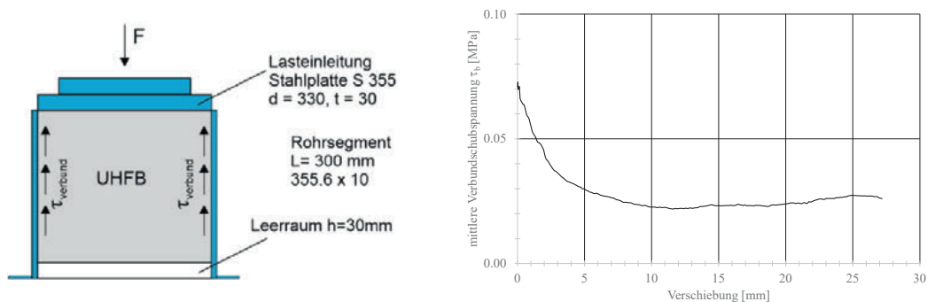
Abb. 4: Pull-Out Versuch an Rohrsegmenten zur Ermittlung der Verbundspannungen
