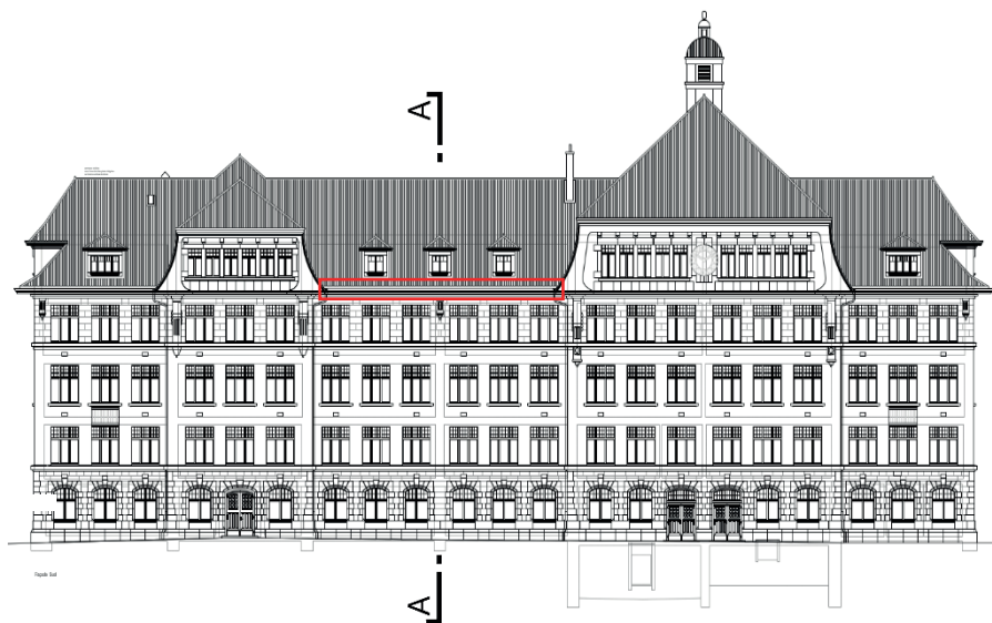
Fig. 1 : Elévation de la façade Sud [1]
