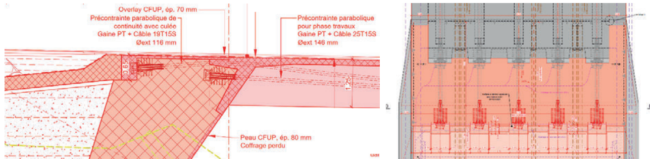
Fig. 11 : Précontrainte – Encastrement blocs de culée
