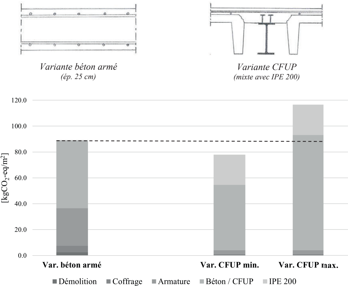
Fig. 16 : Synthèse du bilan carbone des variantes
