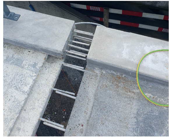
Abb. 19: Fuge nach Einhub
