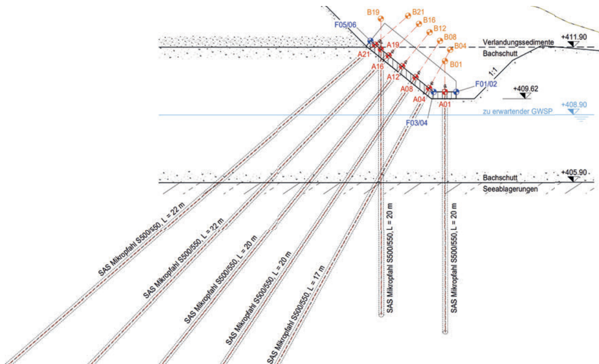
Abb. 12: Schnitt durch die Pfahlfundation
