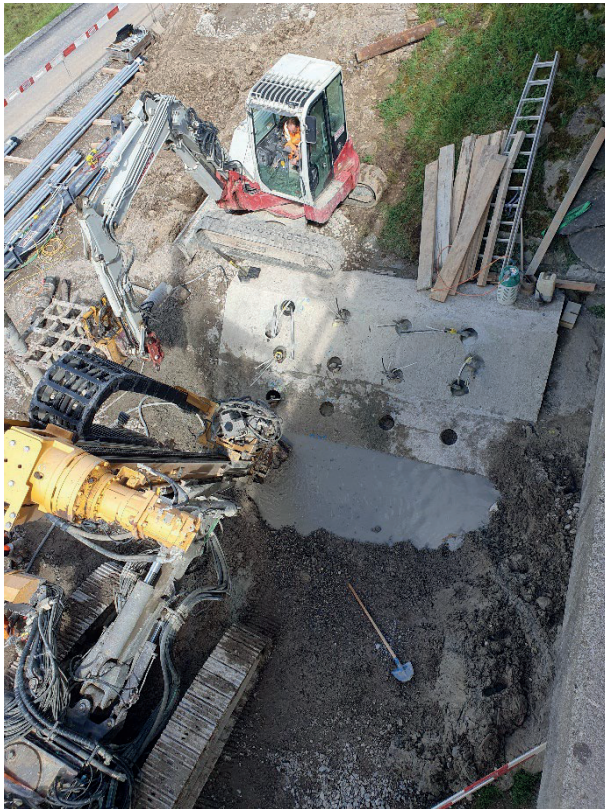
Abb. 13: Mikropfahlfundation
