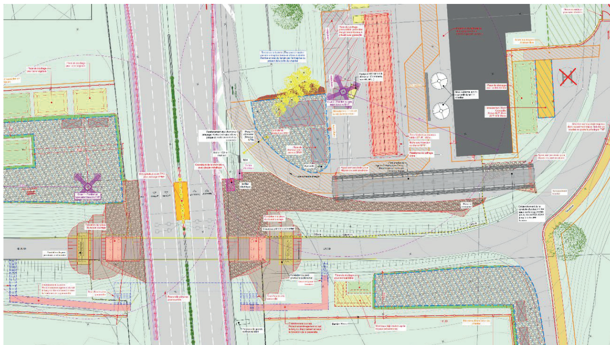
Fig. 16 : Schéma et organisation de la place des installations du chantier
