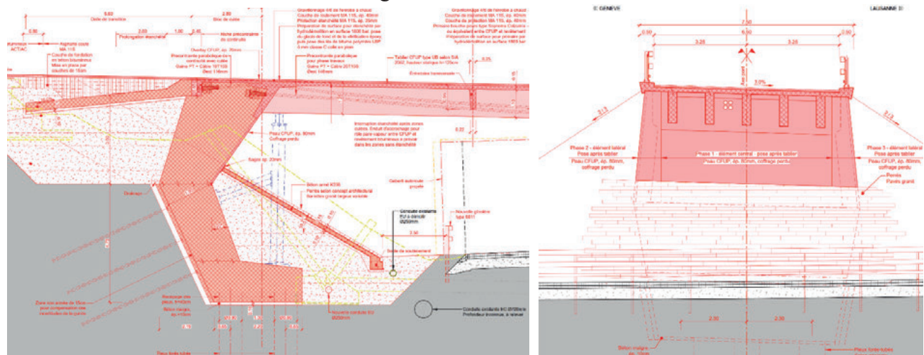
Fig. 12 : Coupe et élévation sur culée
