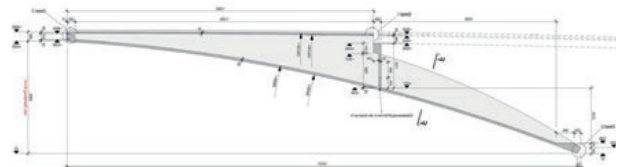
Abb. 15: Bogenelement Seite Altendorf
