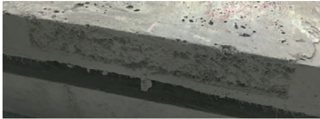
Abb. 26: Querschnitt durch 1. Muster-Elementfuge mit schlechtem Verguss
