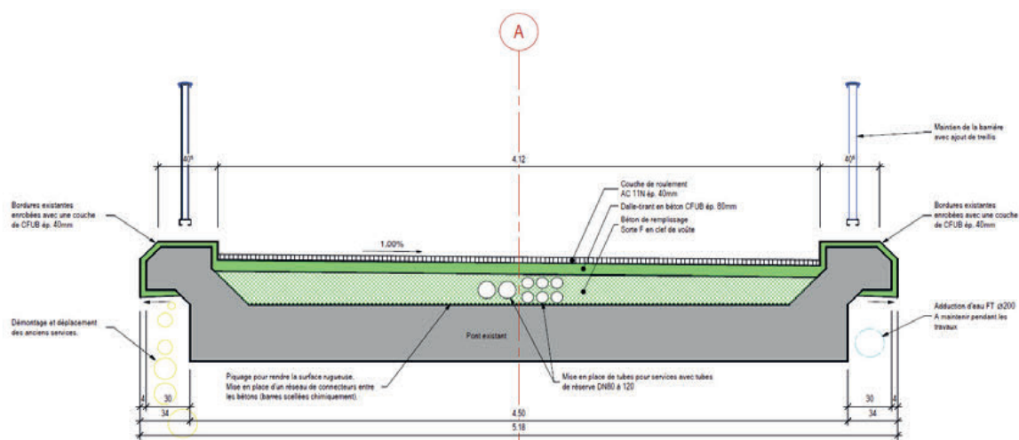
Fig. 2 : Section type du pont avec renforcement CFUP
