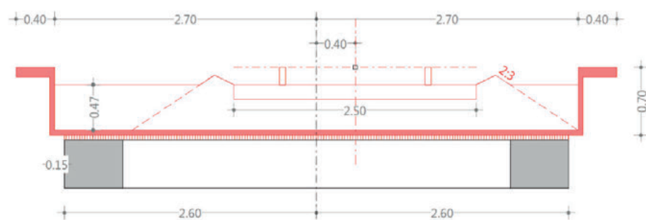
Abb. 6: Idealisierter Querschnitt des UHFB-Schottertrog für die Bemessung
