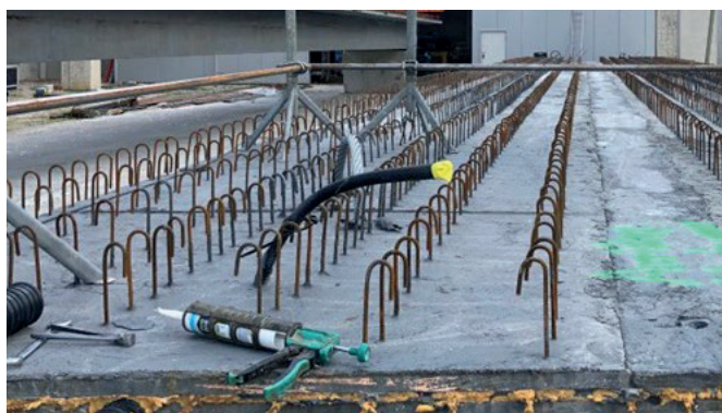
Fig. 7 : Armature de liaison sur éléments CFUP
