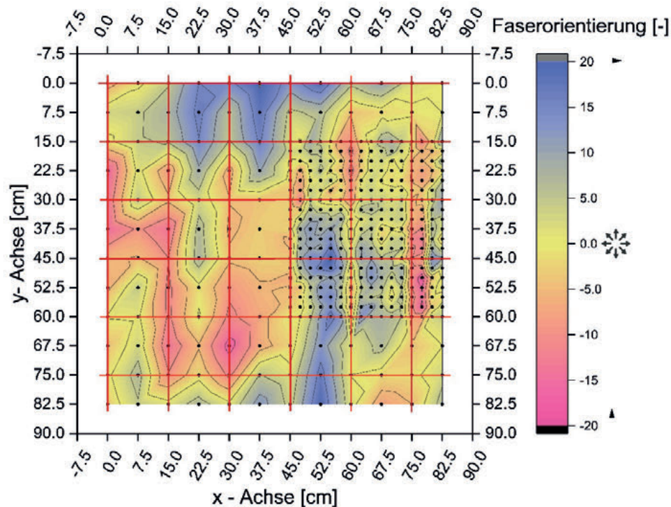
Abb. 8: Verteilung der Faserorientierung im untersuchten Bereich. Farbskala: rot: unidirektionale Faserausrichtung in y-Achse; gelb: isotrope Faserausrichtung; blau: unidirektionale Faserausrichtung in x-Achse. Die roten Linien markieren die Lage der Bewehrung. Die schwarzen Punkte entsprechen den einzelnen Messpositionen.
