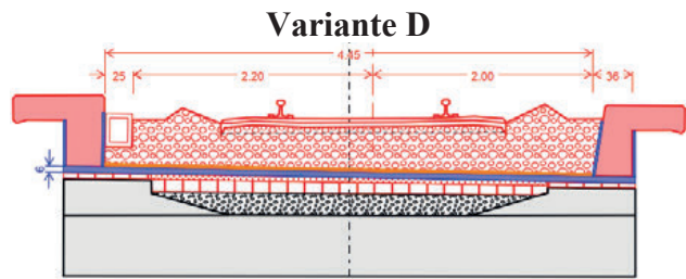
Abb. 3: Querschnitt Variante D: Stahl+Beton-Schottertrog
