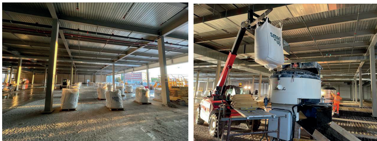
Fig. 7 : Entreposage des big bags sur la dalle du rez-de-chaussée (gauche) et transport du big bag jusqu'au malaxeur (droite)
