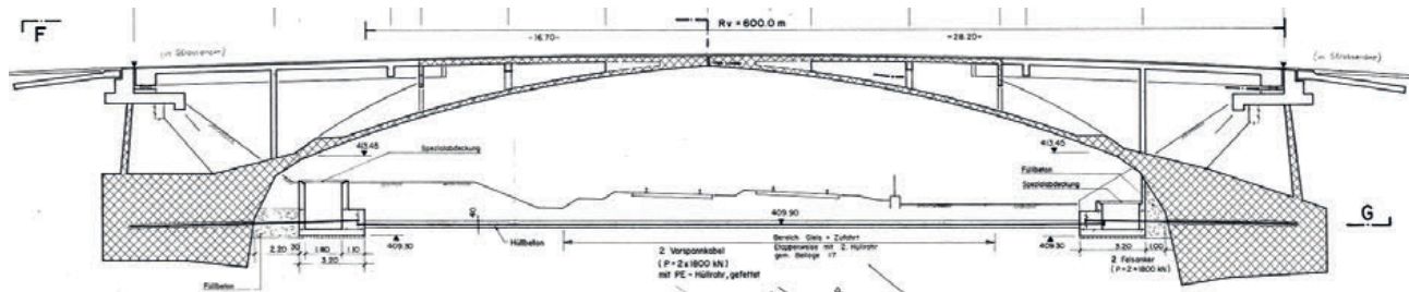
Abb. 2: Längsschnitt einer Maillart-Brücke, Vorspannkabel sichtbar. Gezeichnet 1994, SBB Planarchiv
