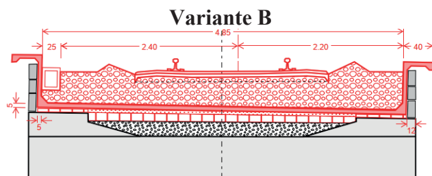
Abb. 4: Querschnitt Variante B: UHFB-Schottertrog innenliegend
