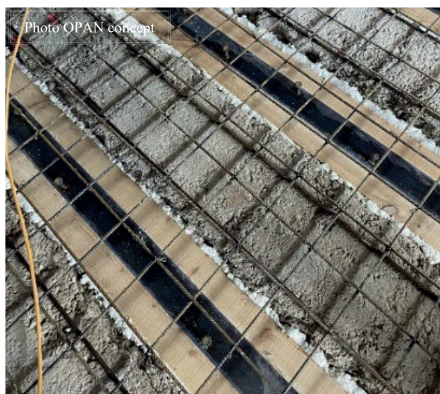
Fig. 8 : Surface supérieure de la dalle avant la mise en œuvre du CFUP
