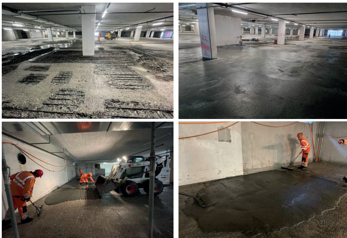
Fig. 11 : Mise en place du CFUP de reprofilage sur la dalle du parking
