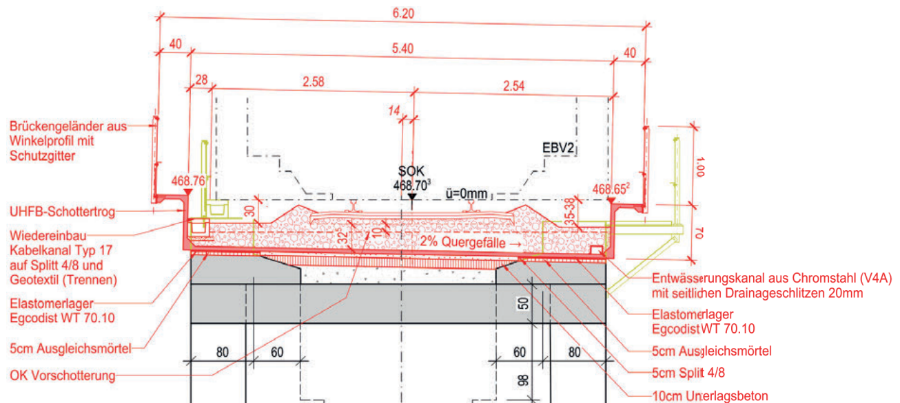
Abb. 29: Querschnitt mit UHFB-Schottertrög (Ausführungsplan Objekt 5 DU Grosshusmatt)
