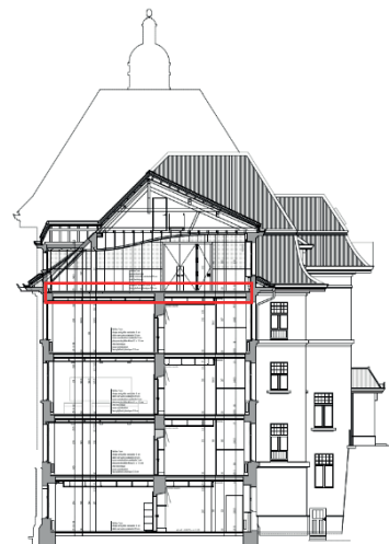
Fig. 2 : Coupe A-A [1]
