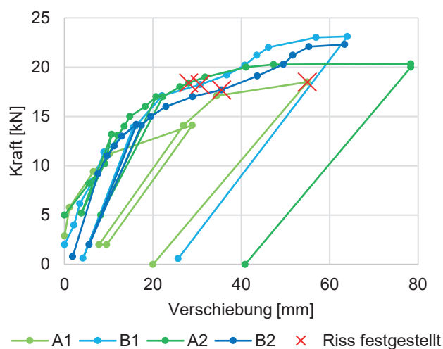
Abb. 13: Kraft-Weg-Diagramme der Belastungsversuche am Randbord des Musterelements
