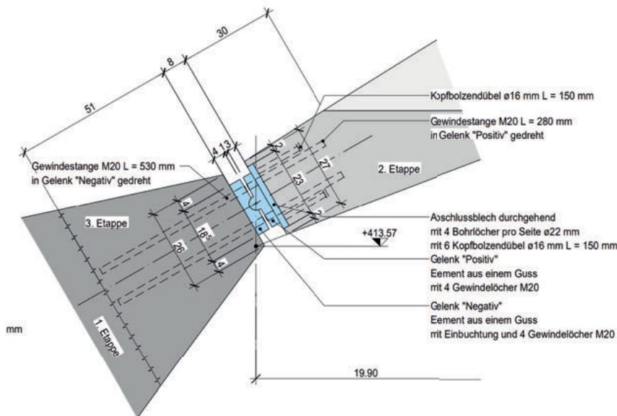
Abb. 10: Kämpfergelenk Detail
