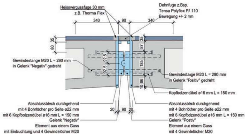
Abb. 8: Scheitelpunkt Detail
