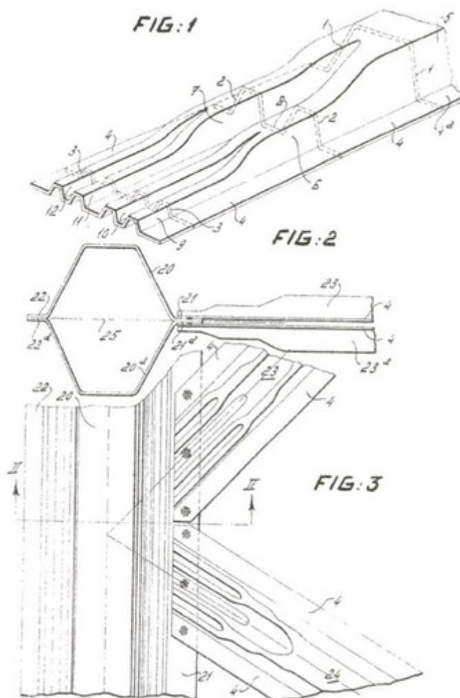
Détail d'assemblage NV Polynorm, 1953(OFFICE EUROPÉEN DES BREVETS)
